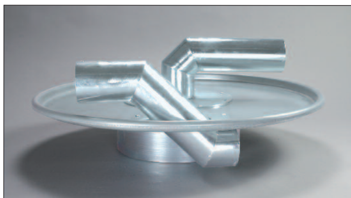
Крышка сепаратора, нержавеющая сталь, для контейнера с сепаратором 50 л/70 л 200 л 50/50 мм - арт. №: 39727 50/50 мм - арт. №: 10856 70/70 мм - арт. №: 10852 70/70 мм - арт. №: 39864 100 л 100/100 мм 50/50 мм - арт. №: 10853 арт. №: 21131 70/70 мм - арт. №: 10854
