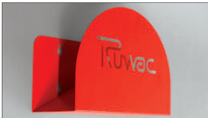
Держатель для шланга, листовая сталь, порошковое покрытие, цвет красный, монтаж на стене Д — 330 мм, Ш — -123 мм, В — 238 мм, вкл. материал для крепления Арт. №: 12080
